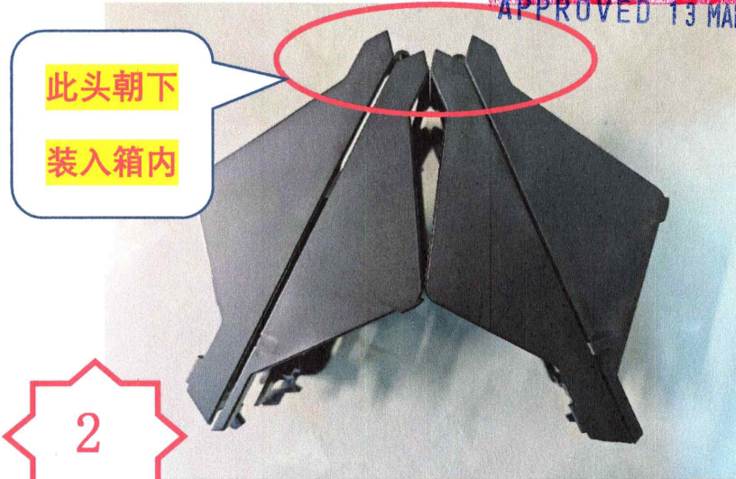
图二，将四个 PA02818 组件如图所示组合
