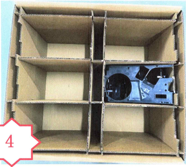
图四，最后再将一个 PA02818 如图放入箱内。 一格装 5 个，一箱共 30 个。
